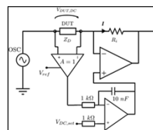
Figuur 18: Meetschakeling met instelbaar DC-niveau (Bauwelinck, 2017)
