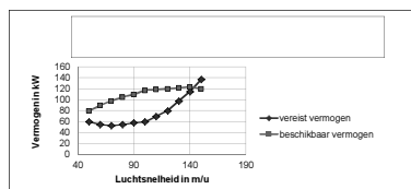
Figuur 8.2: Beschikbaarheid van en eisen aan vermogen lichte vliegtuigen (Smats, 2013)
